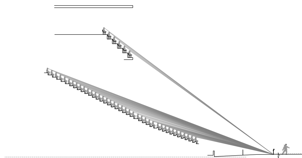
Esquema visibilidad codo Abdon Porte - Atilio García
