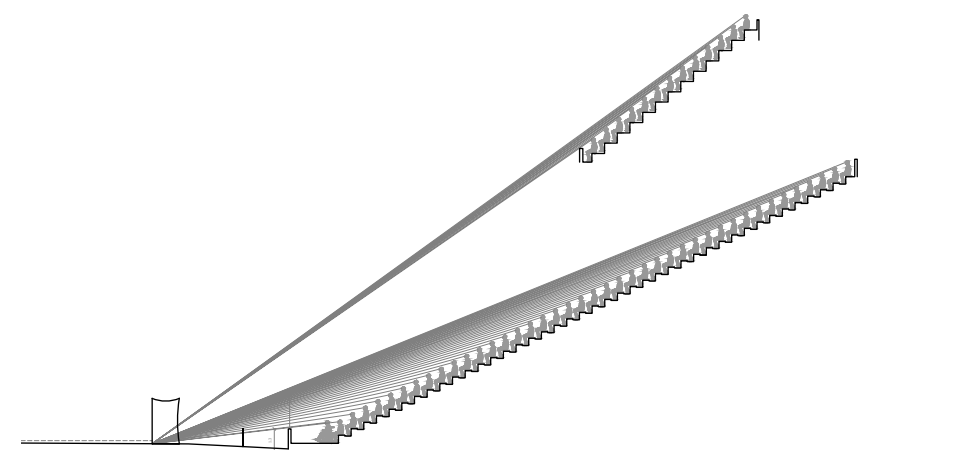
Esquema visibilidad tribuna Héctor Scarone
