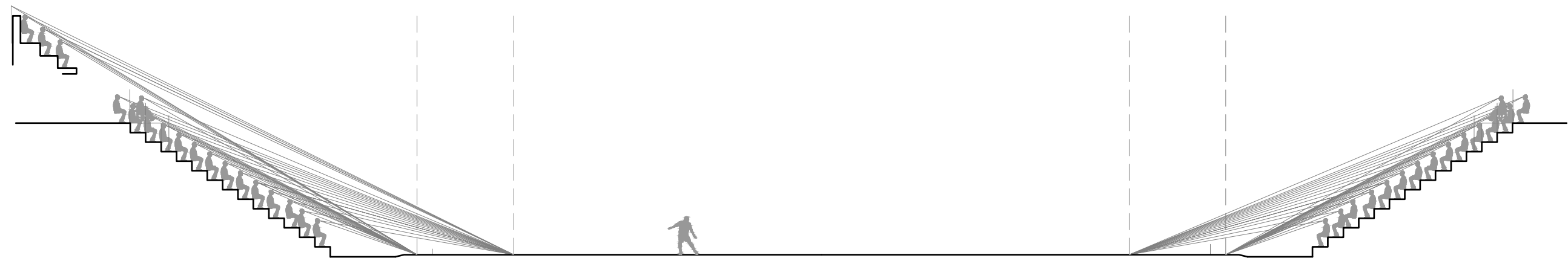
Esquema visibilidad tribuna corte longitudinal
