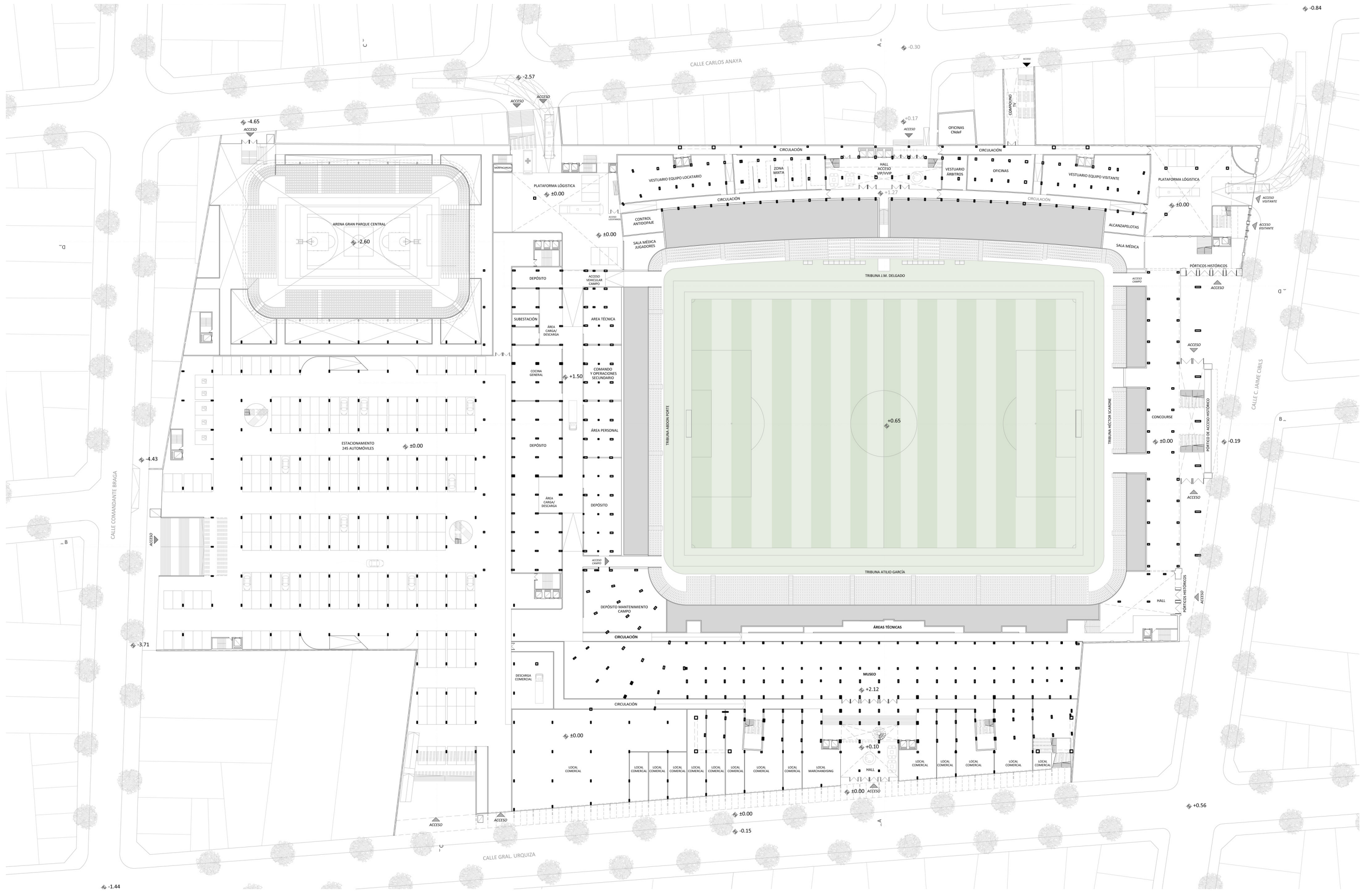
PLANTA BAJA NIVEL 0 | ESC. 1:1000
