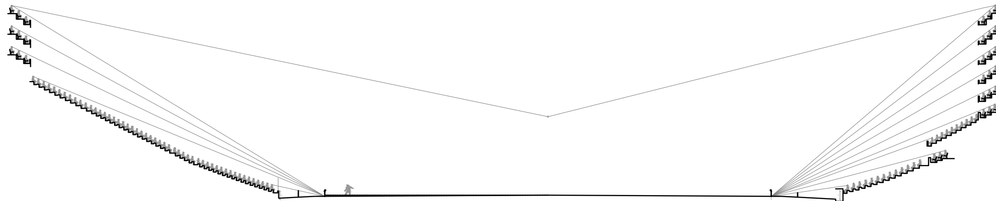
Esquema de visibilidad transversal estadio
