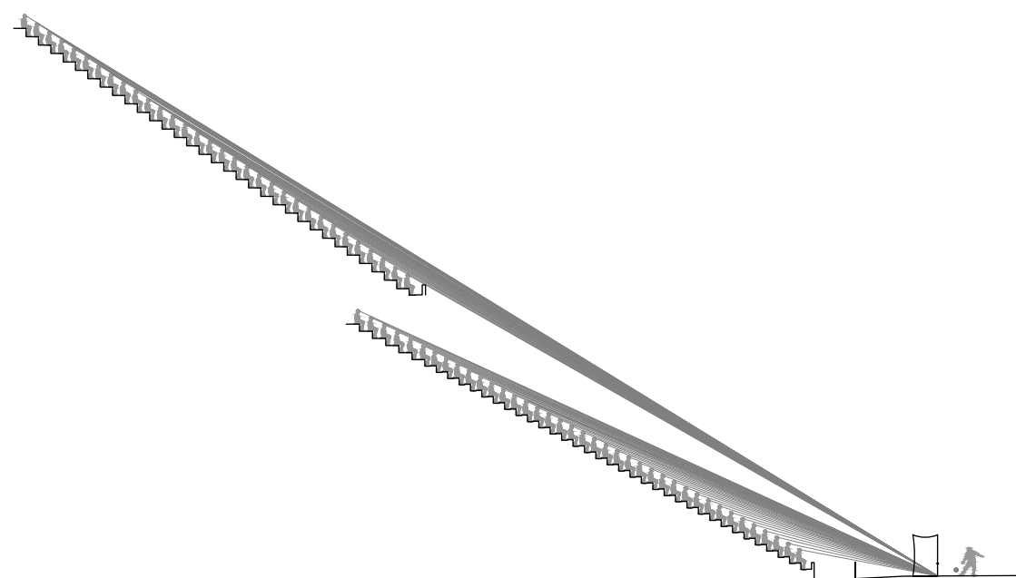
Esquema visibilidad tribuna Abdon Porte
