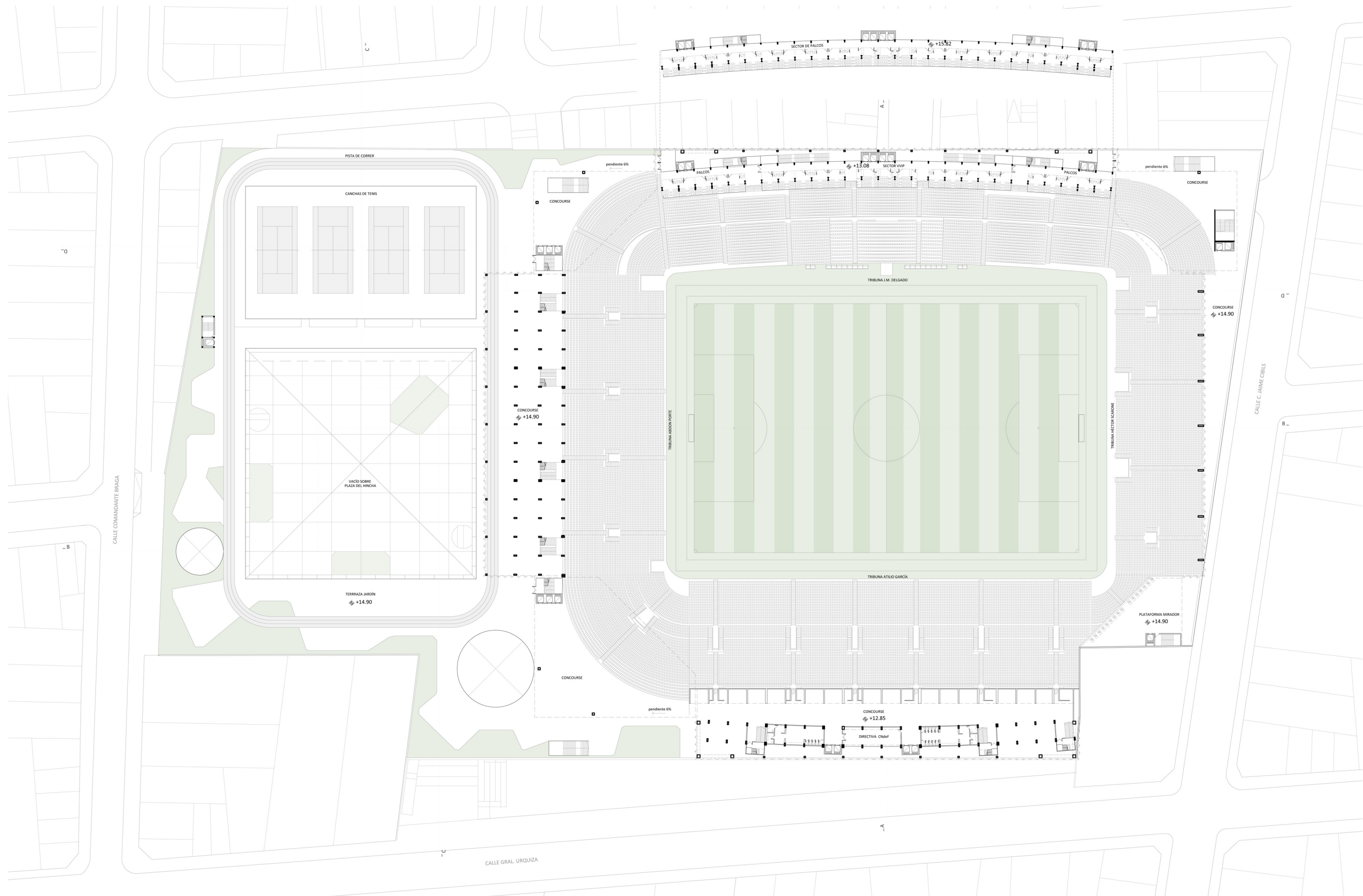
PLANTA NIVEL 4 Y NIVEL 5 | ESC. 1:1000
