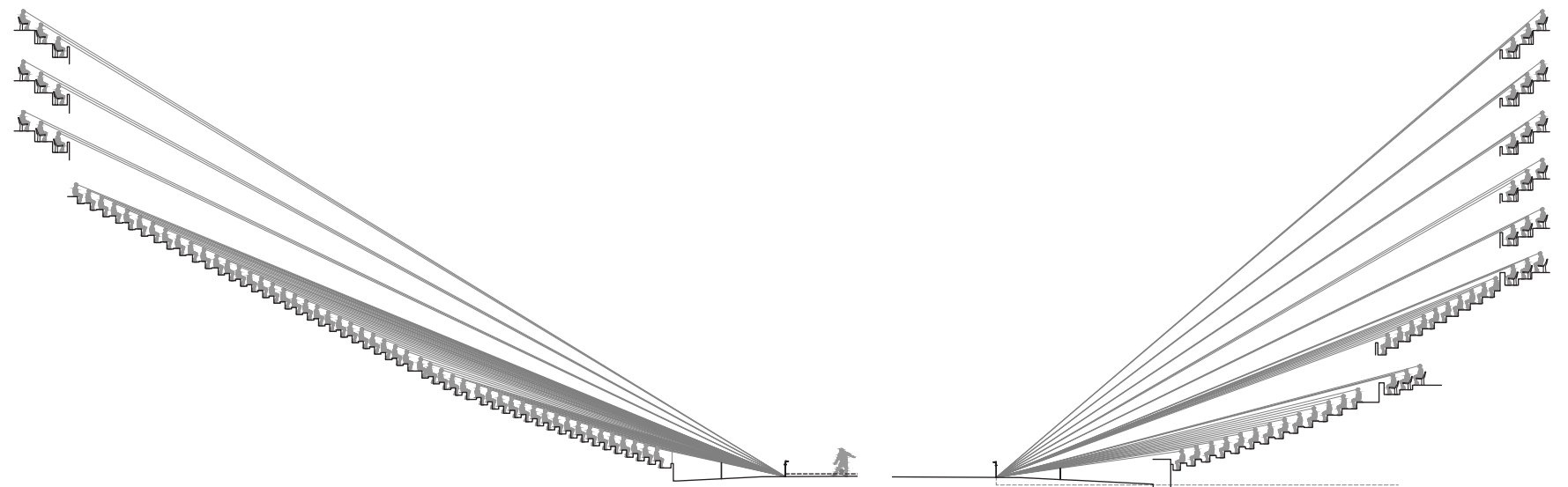
Esquema visibilidad tribuna Atilio García
