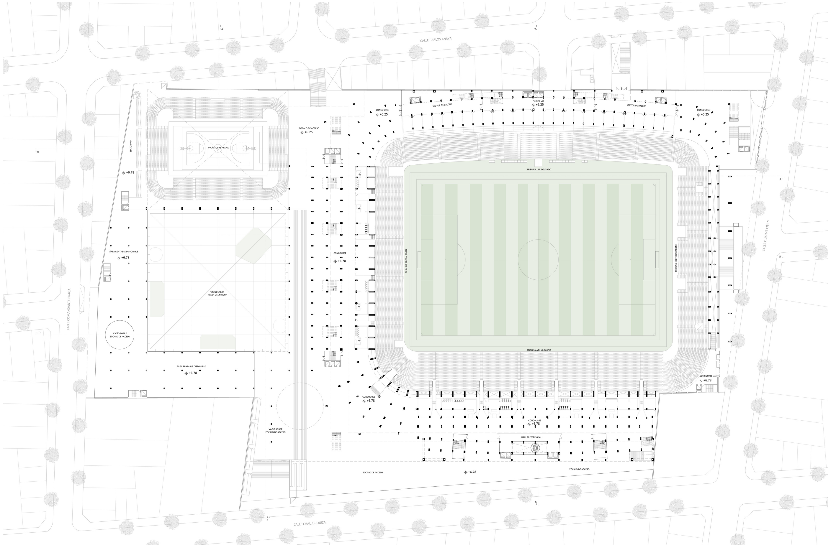
PLANTA NIVEL 2 | ESC. 1:1000
